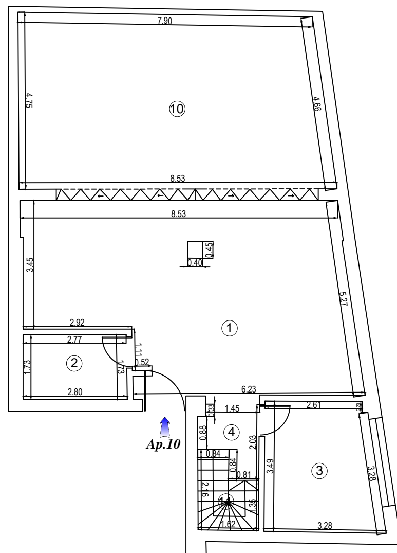
ETAJ 3
